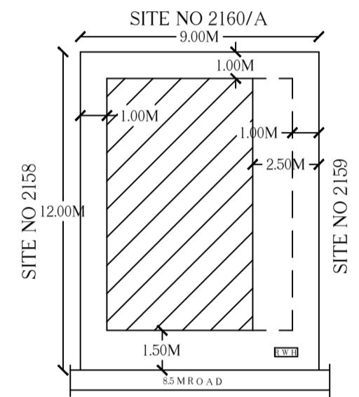
SITE PLAN 1:200
